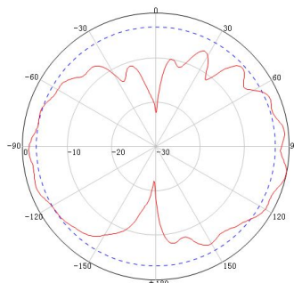
223~235MHz 典型 E 面方向图:
