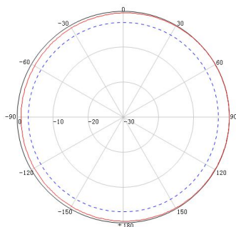
223~235MHz 典型 H 面方向图:
