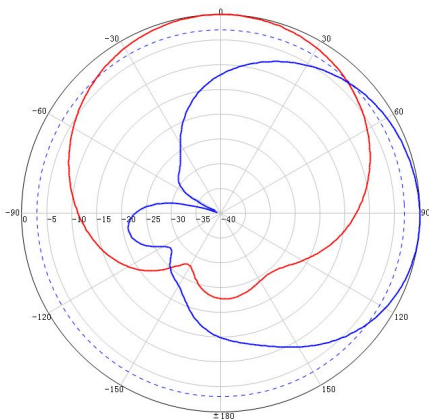
698~800 MHz 典型方向图:
