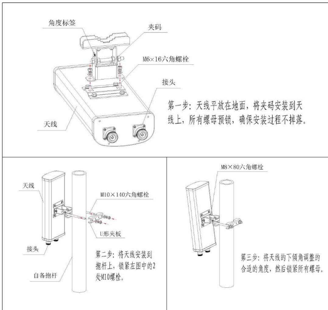
安装示意图
