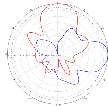
3900~4100 MHz 典型方向图:
