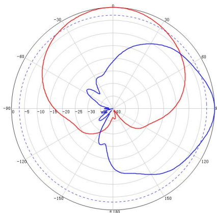
1920~2170 MHz 典型方向图:
