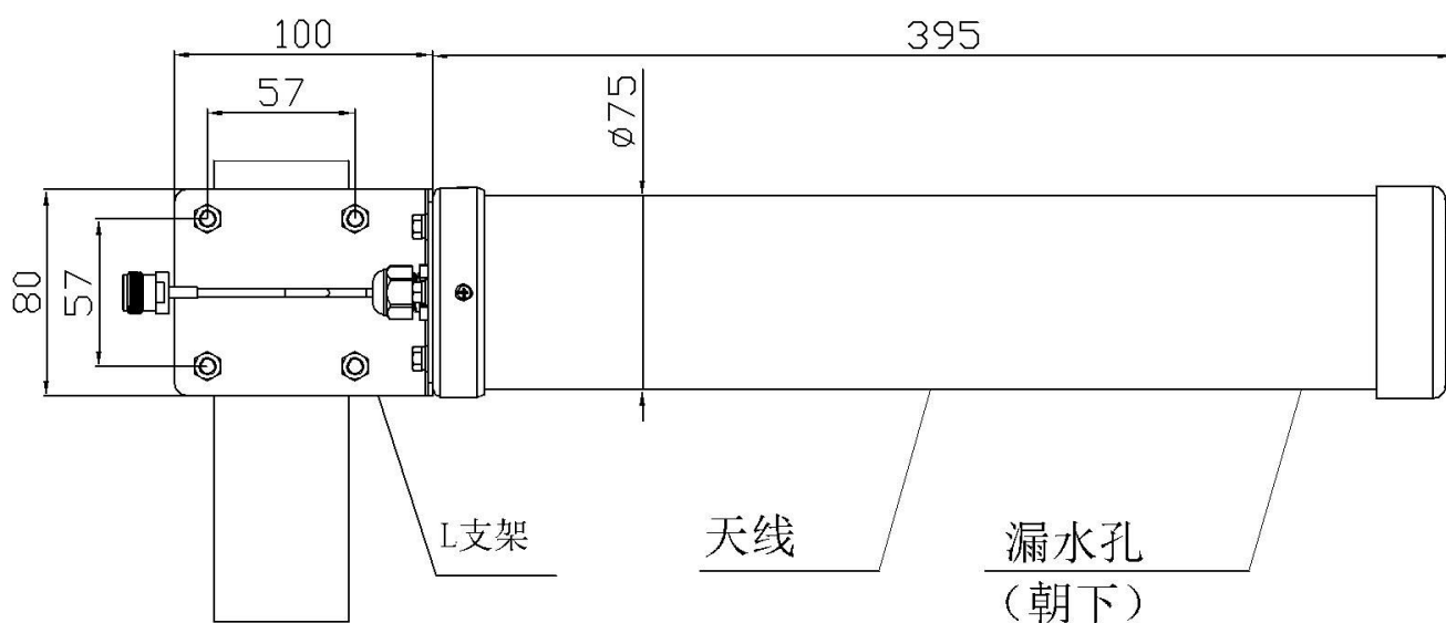
抱杆安装示意图
