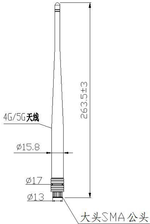
产品尺寸图
