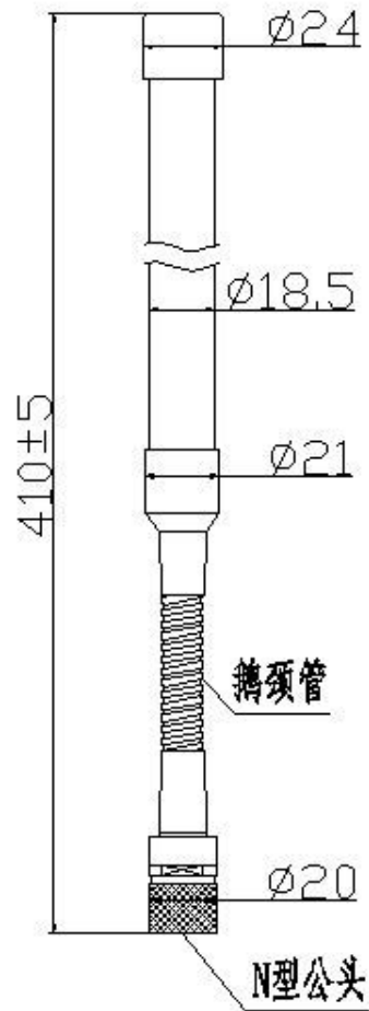
产品外形尺寸图
