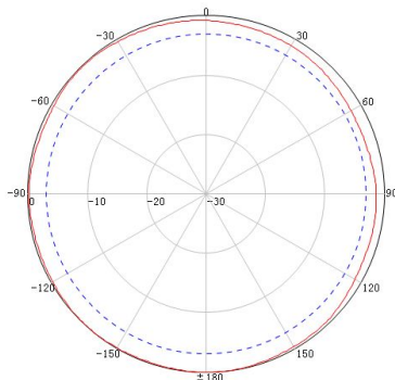
5150~5850MHz 典型 H 面方向图:
