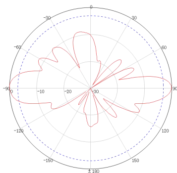
5150~5850MHz 典型 E 面方向图:
