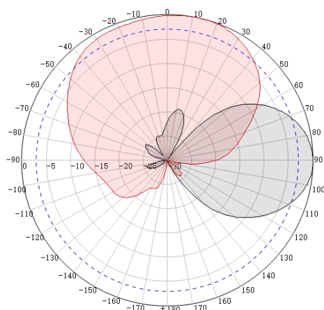
2.4GHz 参考方向图（垂直极化时）
