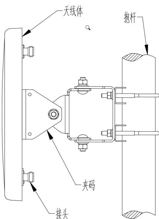
抱杆安装
