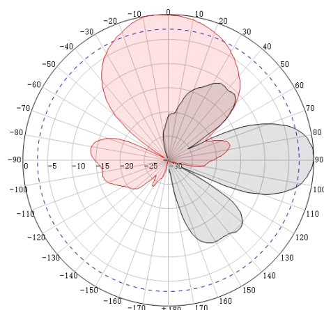
5/6GHz 参考方向图（垂直极化时）
