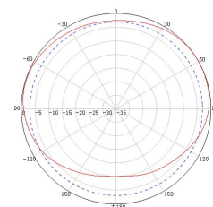
H-面:增益 8.5dBd 3/8 波长, 从塔的间距
