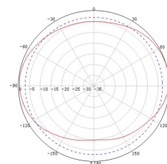
H-面:增益 9.1dBd 1/2 波长, 从塔的间距
