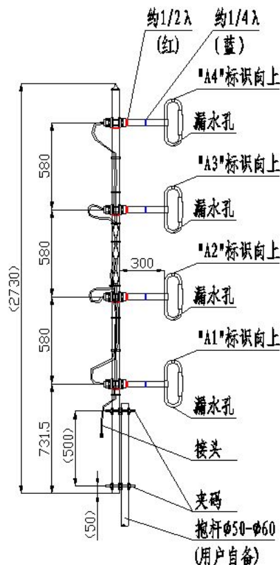
安装示意图
