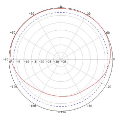
H-面:增益 9.1dBd 1/4 波长, 从塔的间距
