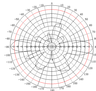
5GHz E 面
