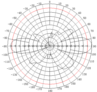
2.4GHz E 面
