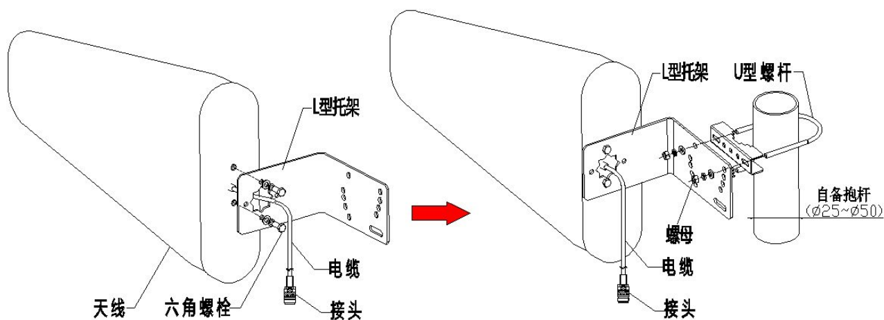
安装示意图
