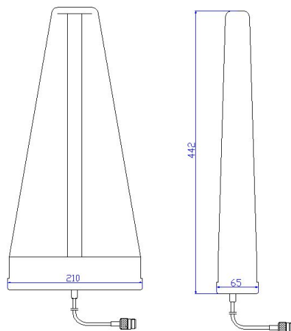
产品尺寸
