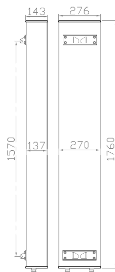
产品尺寸图
