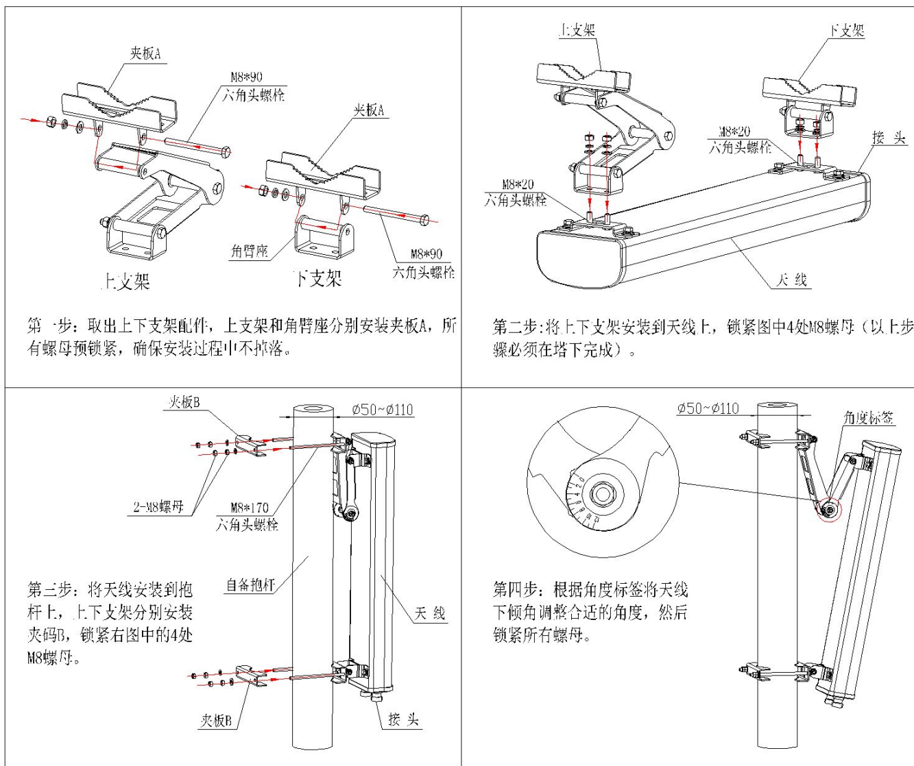
安装示意图
