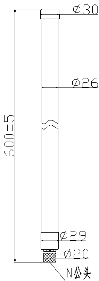
产品外形尺寸图
