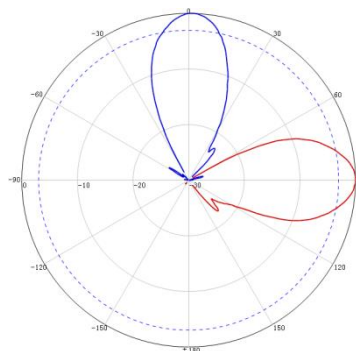
3300-3600MHz: ±45° 极化
